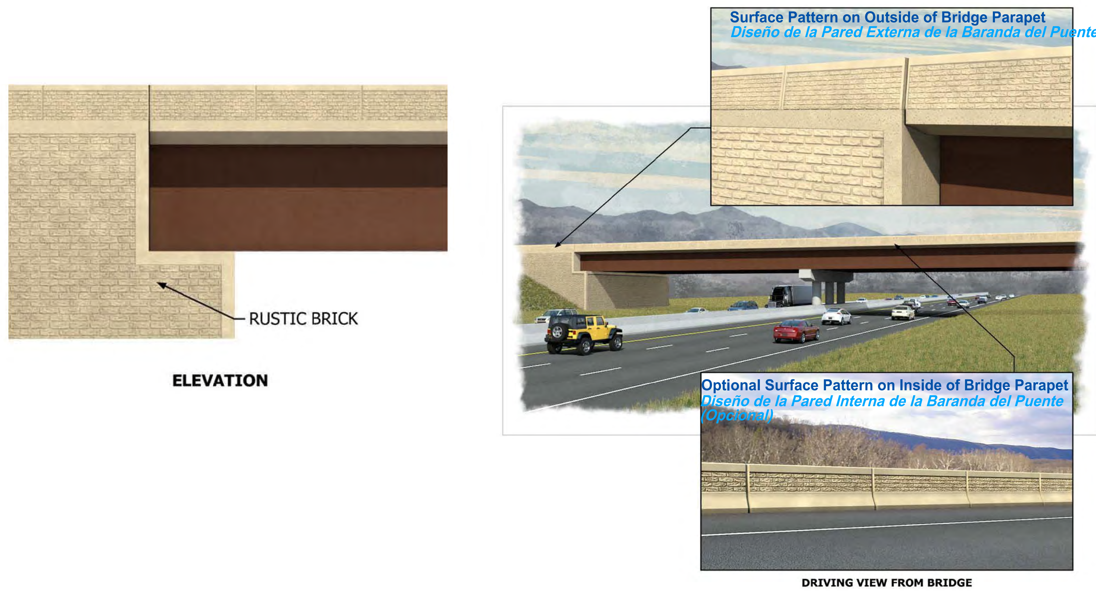
"Rustic Brick" Surface Pattern Option Opción de Diseño de Pared "Ladrillo Rústico"
